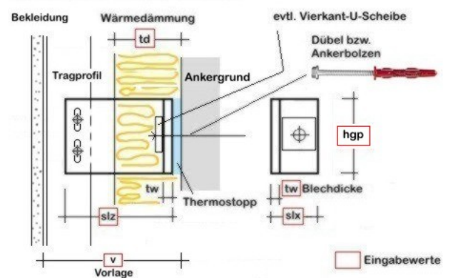
Konsole Gleitpunkt (GP) Tragprofil Bohrschraube/Niete in Langloechern
