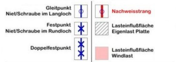
Symbole DynGrafik Tragprofil
