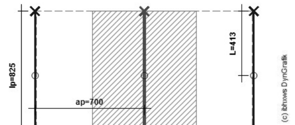
Dummy-Darstellung Tragprofile
